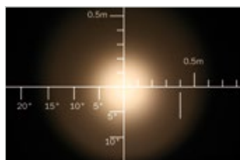
14° Narrow Reflector
