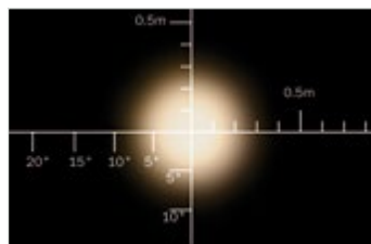
14° Narrow Reflector - Glare Control
